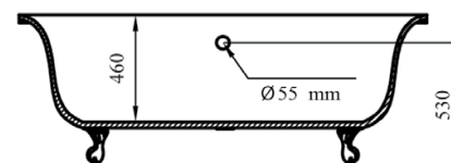
SEÇÃO AA
